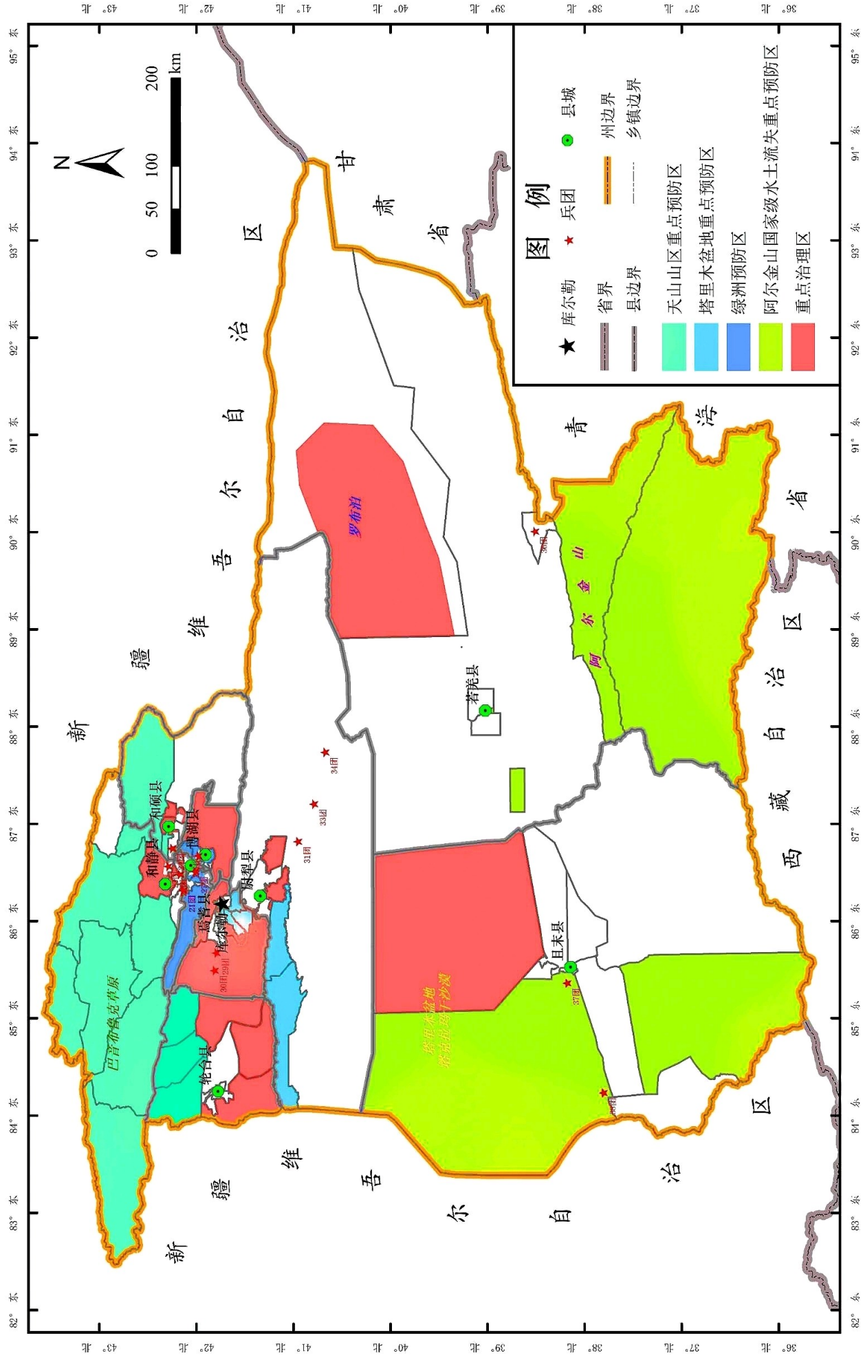
附件2 巴音郭楞蒙古自治州水土流失重点预防区、重点治理区分布图
